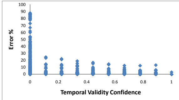
Fig. 10: Reported Confidence vs. Actual Error
